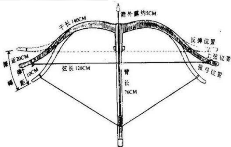
秦弩的弓形变
